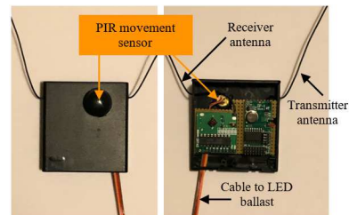
Fig. 7. Detector prototype.
