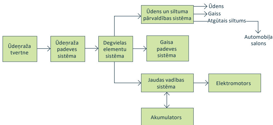
6.1. attēls. FCEV darbības princips.
